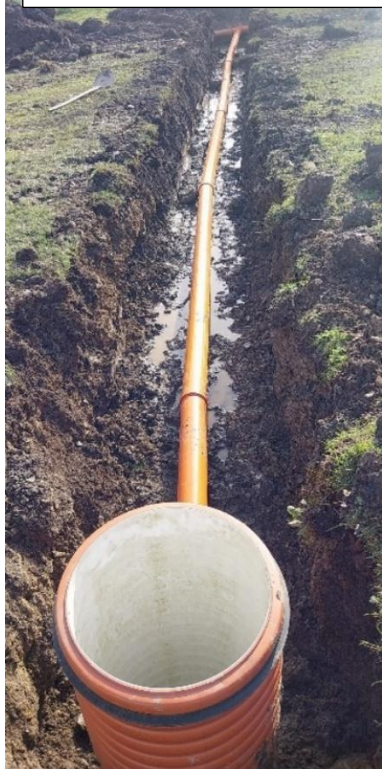
Odvodnění parkoviště – fotbalový areál
